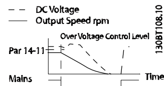
Рисунок 3.35 Управляемое замедление, более длительное размыкание цепи. Замедление длится до тех пор, пока в системе остается энергия, после этого двигатель останавливается выбегом.
