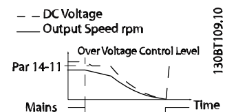
Рисунок 3.37 Кинетический резерв, более длительное замыкание сети. Двигатель останавливается выбегом, как только энергия в системе падает слишком низко.
